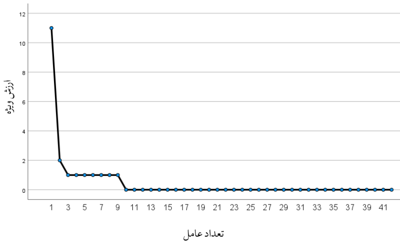
نمودار ۱: نمودار اسکری پلات برای تعیین تعداد عامل ها
